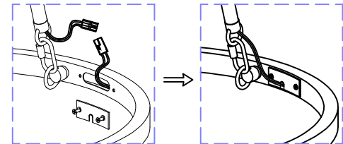
接线方式B
